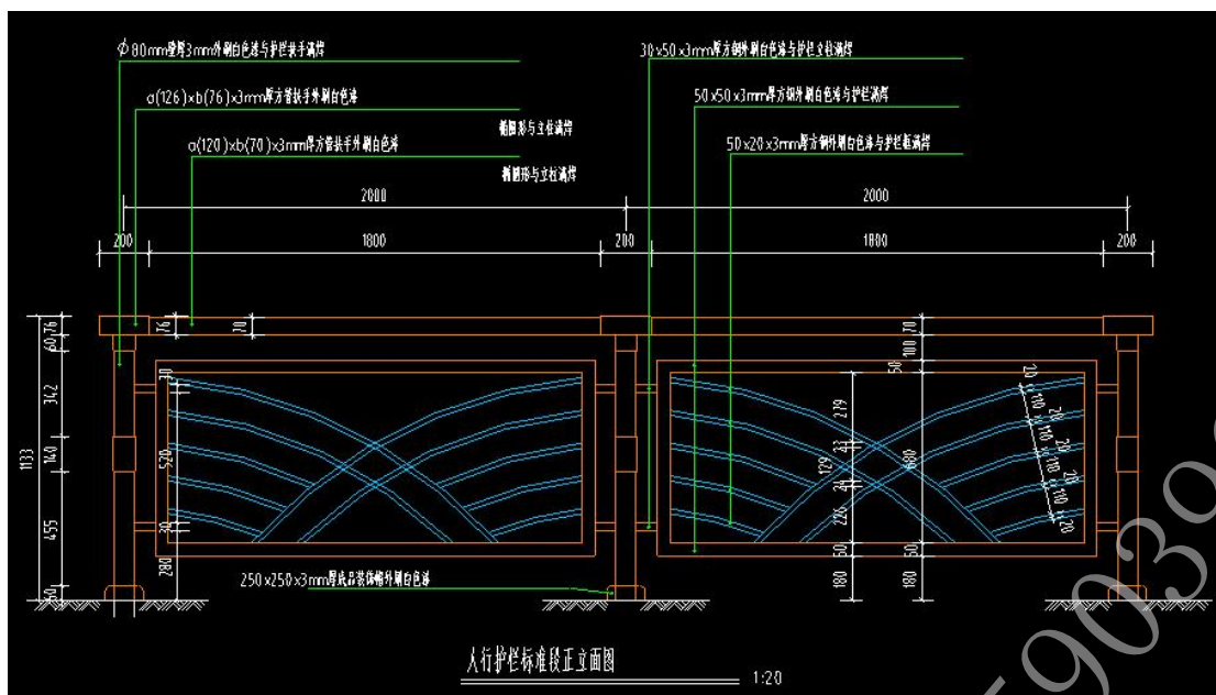
2.4.4. 图纸四：人行道护栏平面图（扶手）
