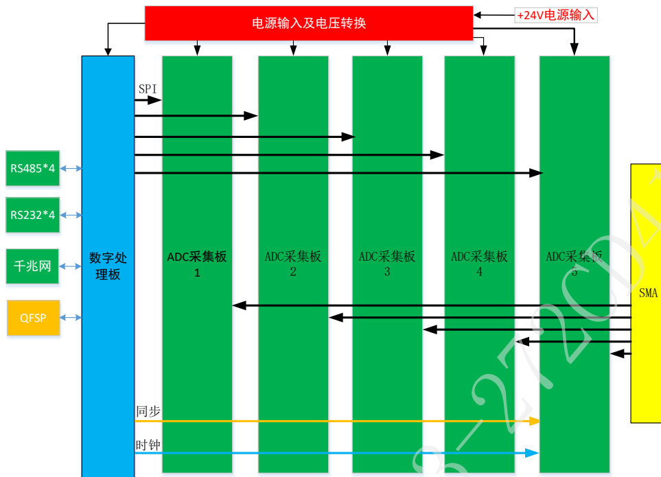
图 1 硬件组成
